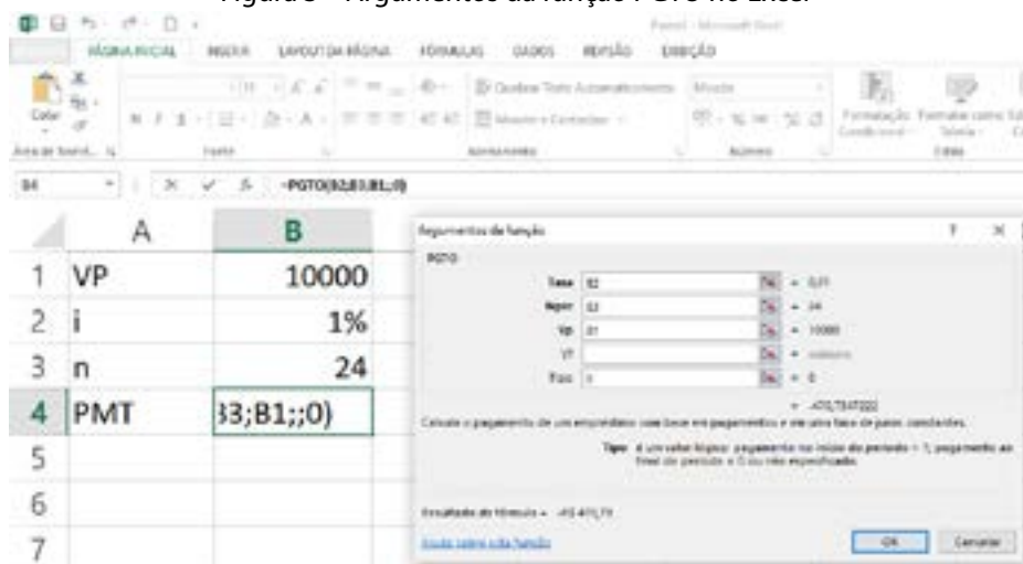
Figura 3 – Argumentos da função PGTO no Excel®
